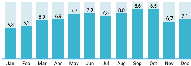
Rasio Pengupasan Lapisan Tanah Penutup Bulanan Monthly Stripping Ratio
